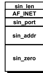
sockaddr_in
