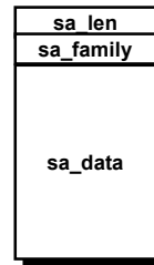
sockaddr
